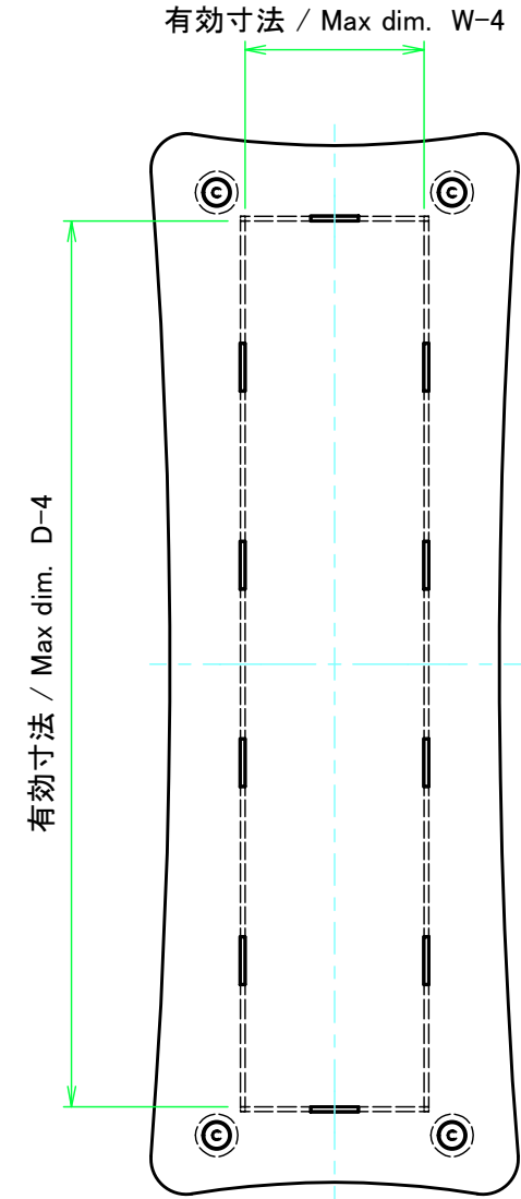
下カバー / Bottom cover
