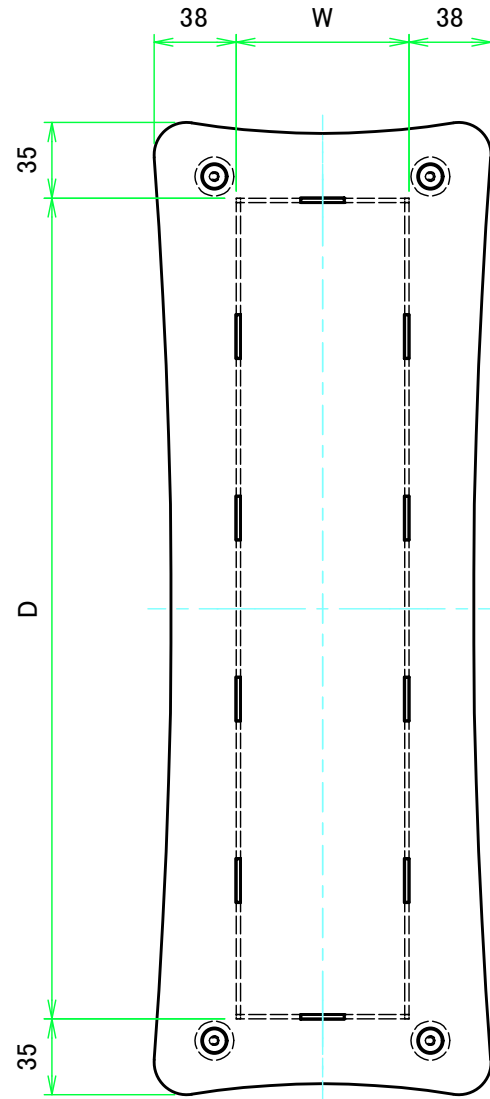
上カバー / Top cover
