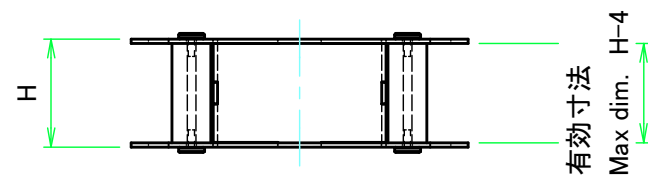
Wパネル1 / W panel 1
